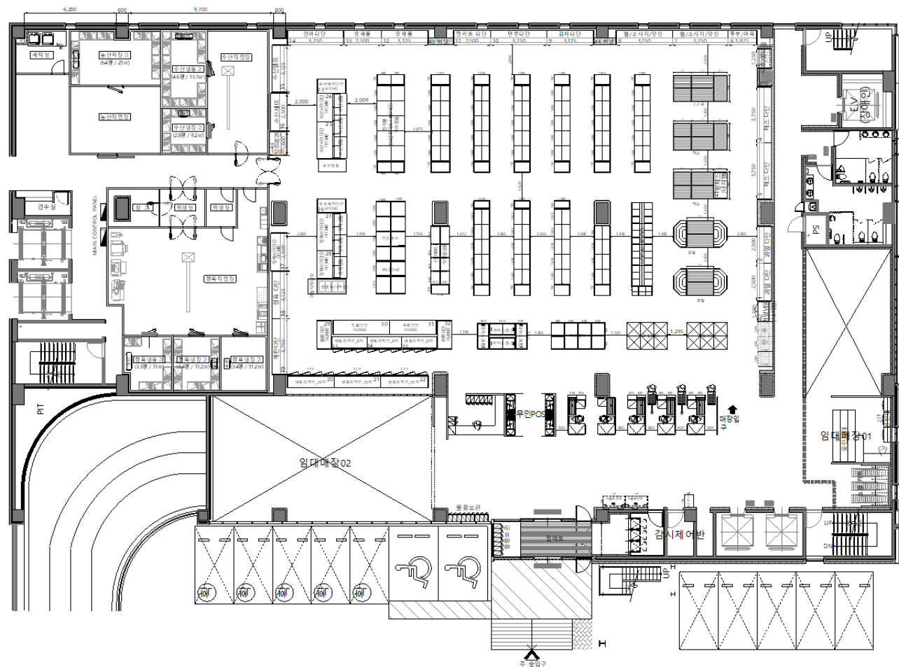
지상 1층 평면도 SCALE: 1/200
