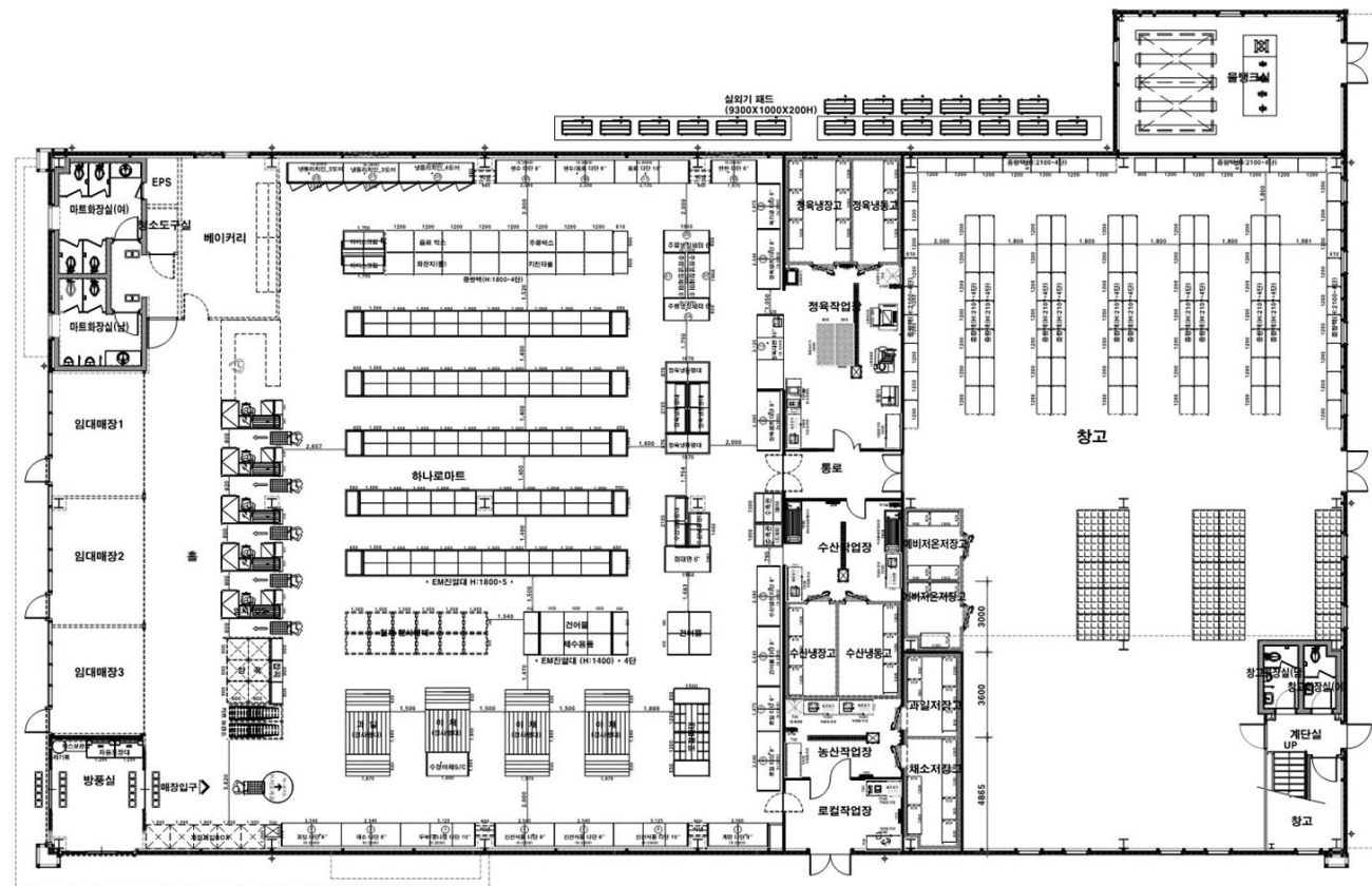
지상 1층 평면도 SCALE: 1/200
