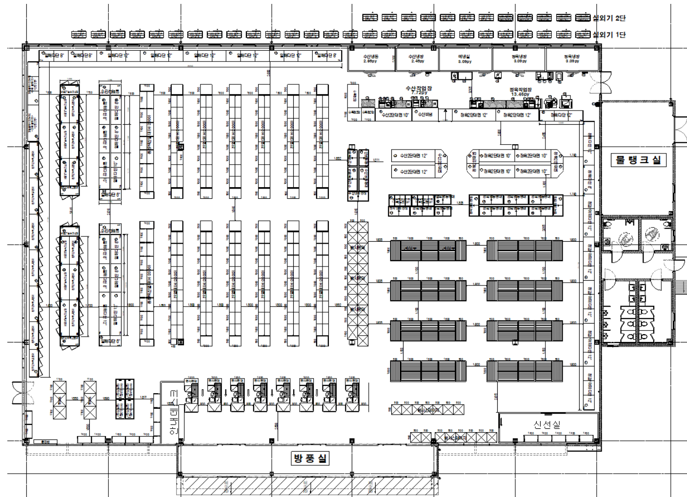
지상 1층 평면도 SCALE: 1/200
